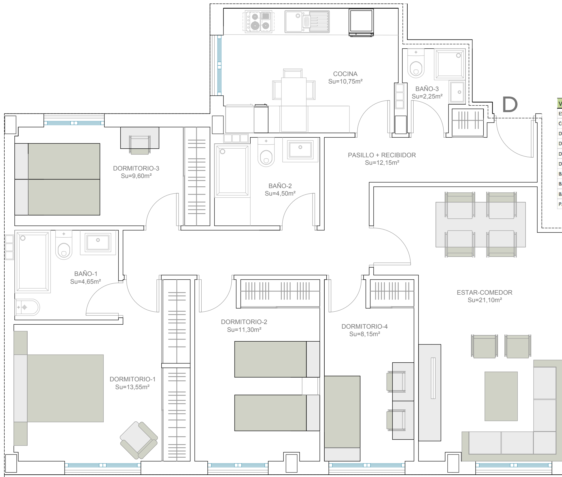
Planta 2 a VIVIENDA D - PORTAL-3 Su=98,00m 2 4 dorm.
