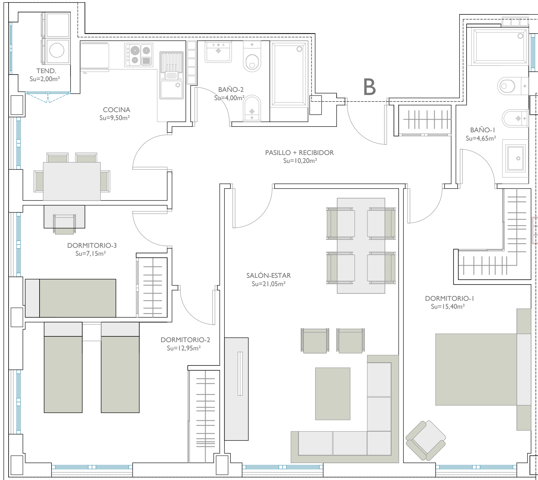
Planta 1ª VIVIENDA B - PORTAL-1 Su=86,90m 2 3 dorm.
